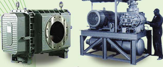
รูทโบลเวอร์และแวนคัมปั้ม (Roots Blower, Vacuum Pump)
